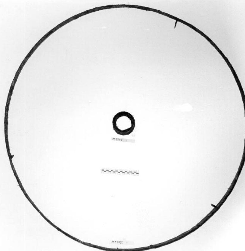
Cerchio e mozzo di ruota di biga in ferro, dall'album della 1ª inventariazione
